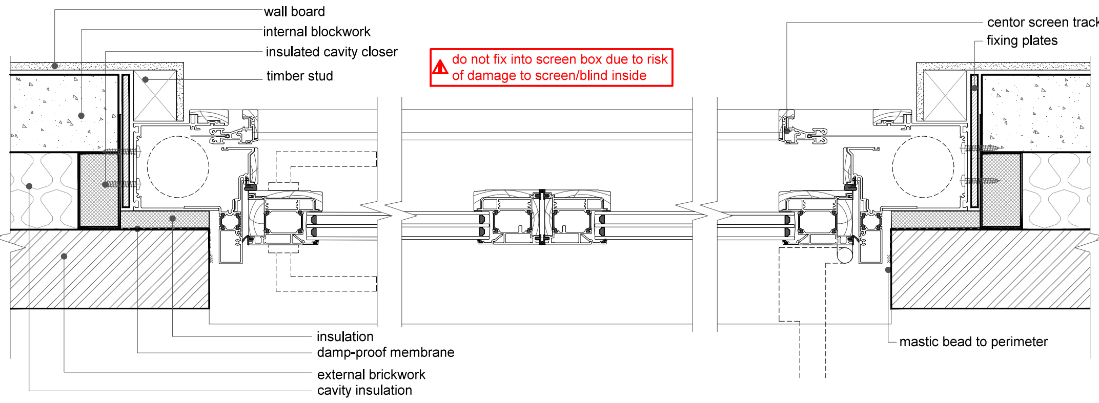
1 jamb detail
